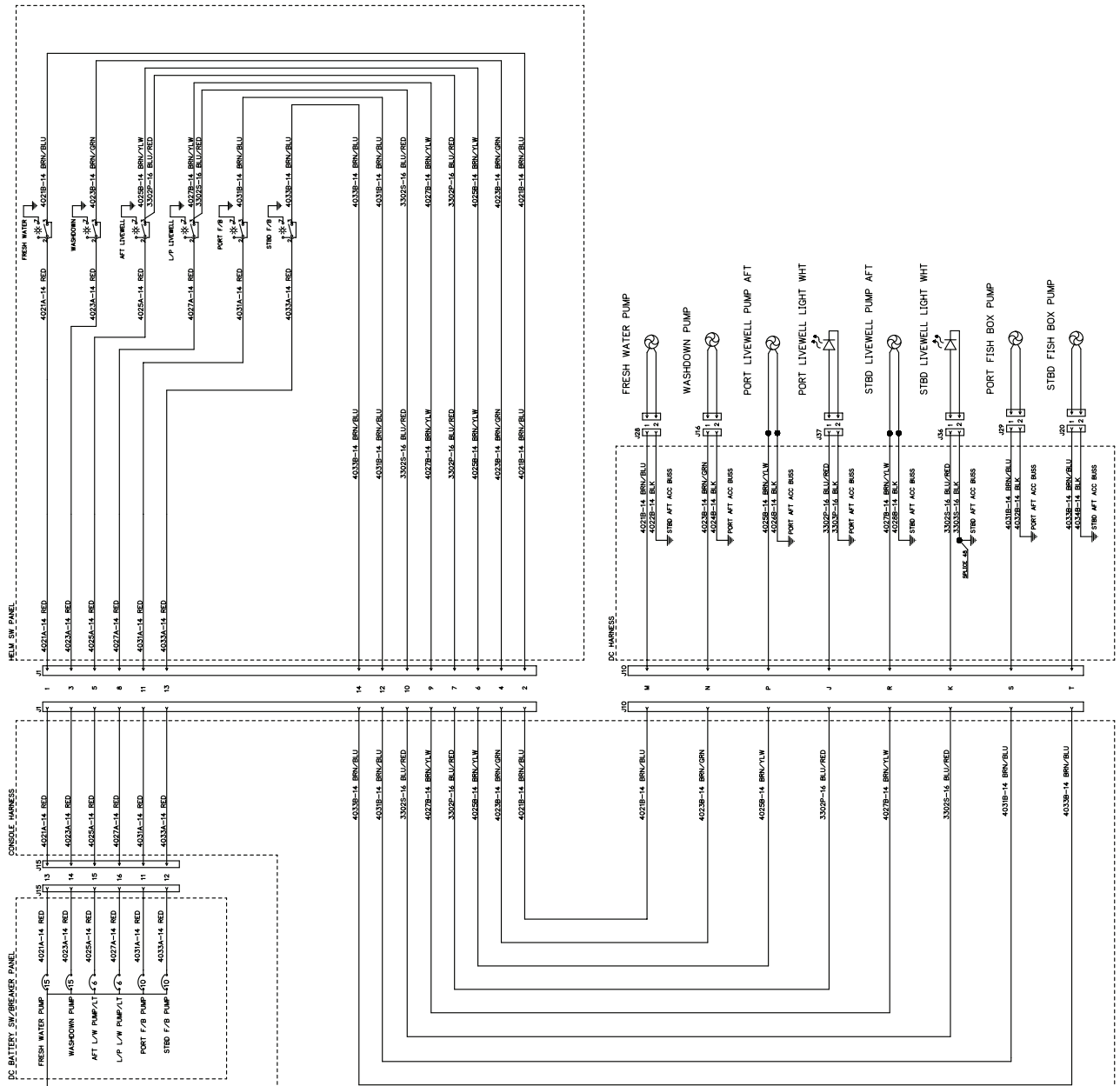
230 Outrage Schematic- Sheet 16 Fig. 4.23.1
